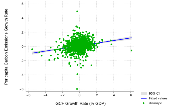
(d) Correlation dlemispc-dlgcf
